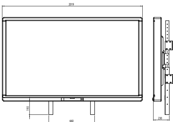
Bottom position / Pozycja dolna: 190 mm
