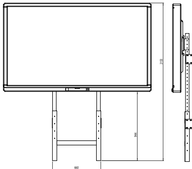
Top position / Pozycja górna: 2193 mm
