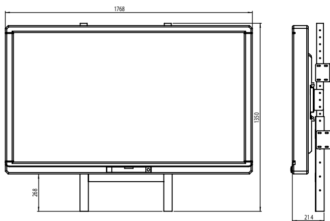
Bottom position / Pozycja dolna: 268 mm
