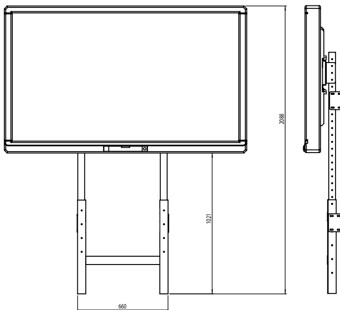
Top position / Pozycja górna: 1021 mm
